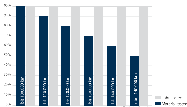
Materialkosten nach Betriebsleistung des beschädigten Bauteils
